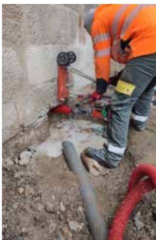
Connexion aux réseaux d'eau dans l'église Sainte-Marie-Madeleine par l'entreprise TPE
